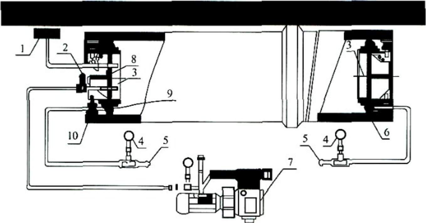
图 E.0.1 排水管道闭气检验装置图
