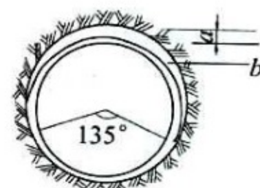
图 6.3.7 超挖示意图
