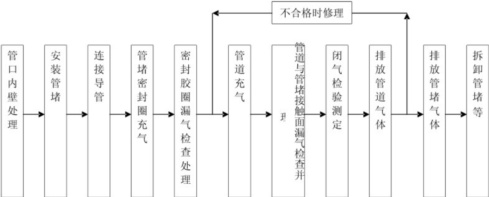
图 E.0.2 管道闭气检验工艺流程图
